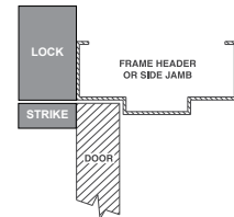
Top Jamb Inswing or Sliding Door
