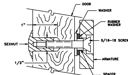
FIG. 2B SOLID DOOR
