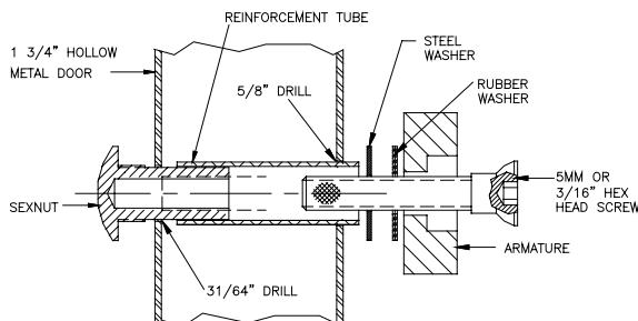
FIG. 2A HOLLOW METAL DOOR
