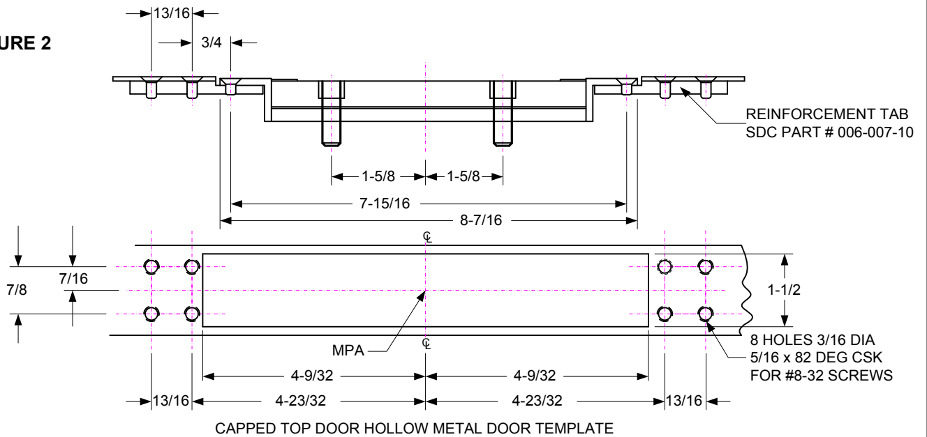
CAPPED TOP DOOR HOLLOW METAL DOOR TEMPLATE
